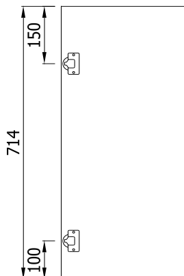
Fasādes grīdas skapjiem ar izlietni
